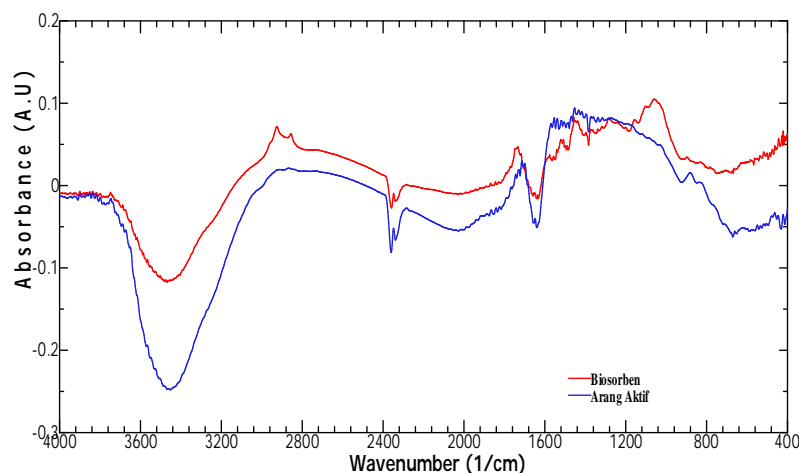
Gambar 1. Analisis gugus fungsi biosorben dan arang aktif sebelum proses adsorpsi menggunakan FTIR
