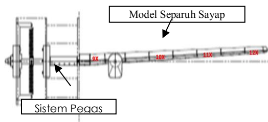
Gambar 6. Gambar instalasi model separuh sayap pesawat N219 dan sistem pegas di terowongan angin.
