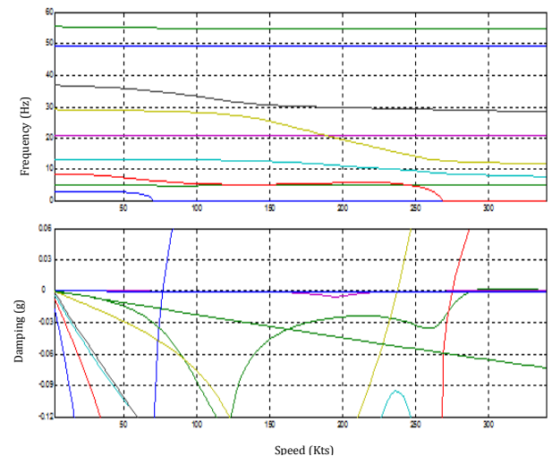
Gambar 7. Kurva V-g-f Model Uji Akhir Pegas Sedang hasil NASTRAN
