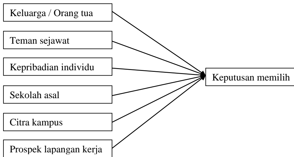
Gambar 1. Model Analisis Data dengan Regresi Linear Berganda
