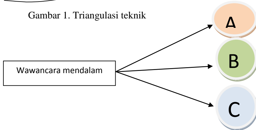
Gambar 2. Triangulasi sumber
