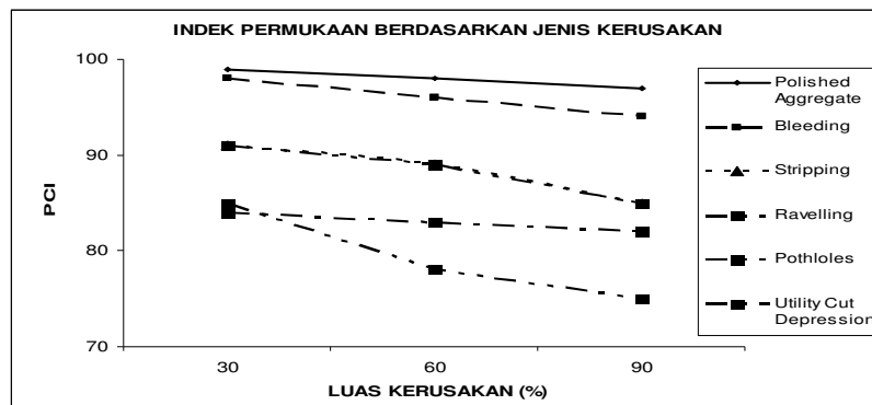
Gambar 4.1 Indeks Permukaan Berdasarkan Jenis Kerusakan
