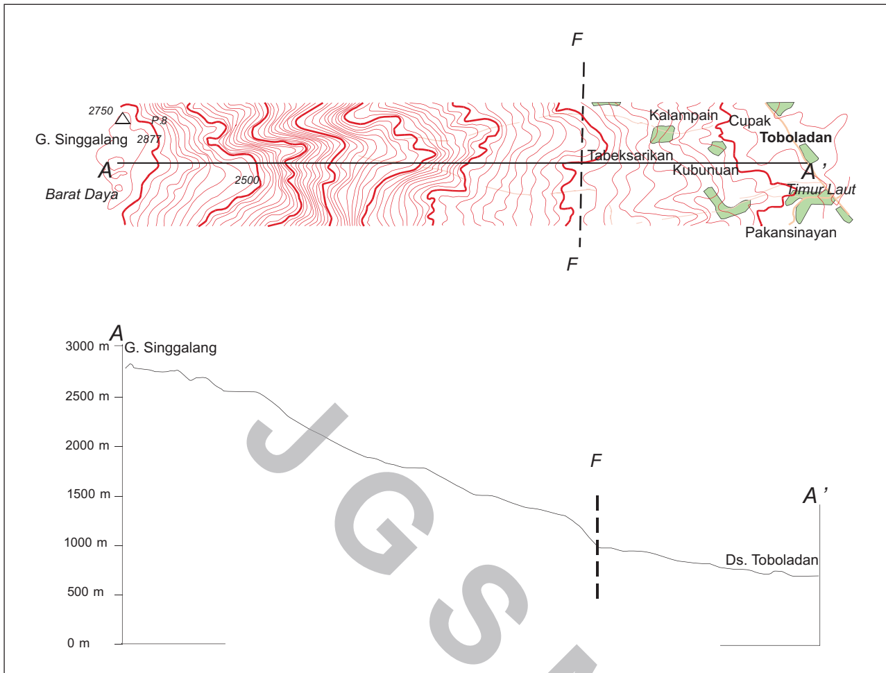
Gambar 8. Profil lereng kaki timur laut Gunung Singgalang, sudut kemiringan lerengnya sangat dipengaruhi struktur sesar Sumatera, arah potongan penampang (A-A') N37°E.
