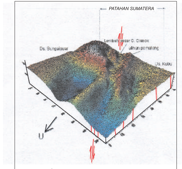
Gambar 15. Cerminan tiga dimensi bentuk lahan tektonik di sekitar Sungai Puar-Kubu, tersusun oleh batuan piroklastika Gunung Marapi berumur Kuartar.
