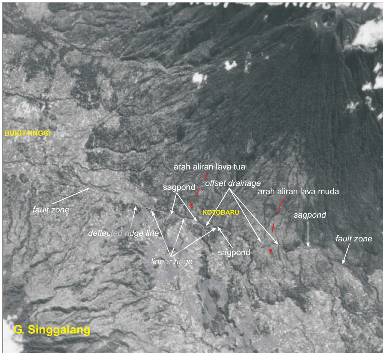
Gambar 4. Penampakan morfologi Gunung Api Marapi-Singgalang berikut elemen morfostruktur daerah Kotobaru dan sekitarnya, terekam dari foto udara tahun 1996.
