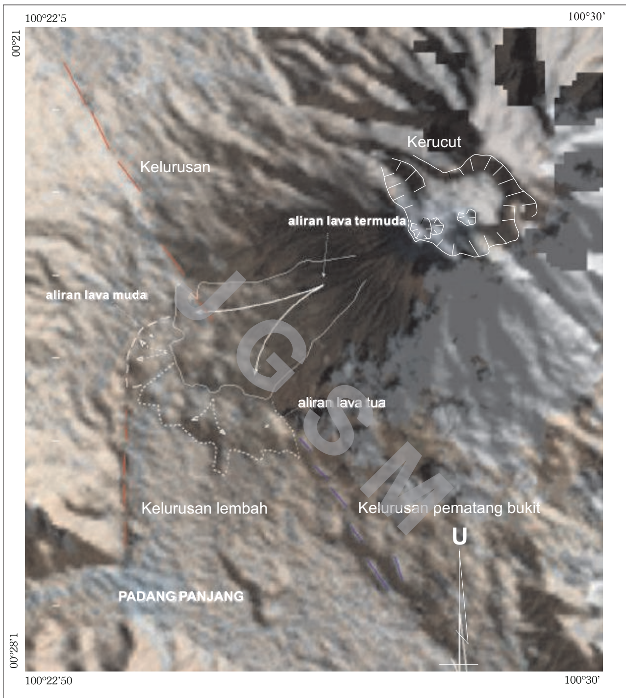
Gambar 6. Cira landsat menunjukkan lereng barat kaki Gunung Merapi yang tersusun oleh lava termuda dan guguran piroklastika, tidak terpengaruh oleh sesar Sumatera.
