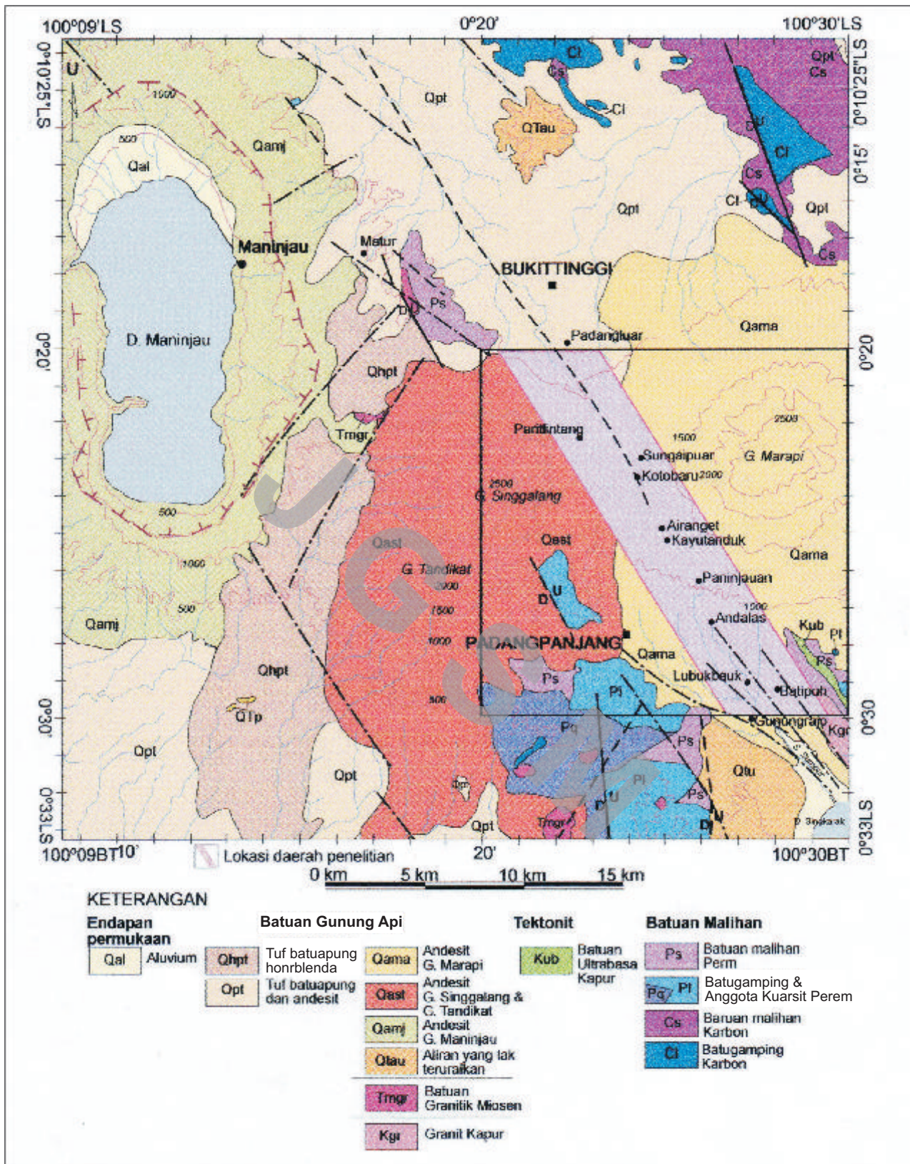
Gambar 2. Peta geologi daerah Padangpanjang dan sekitarnya (dikutip sebagian dari peta geologi lembar Padang skala 1:250.000, oleh Kastowo, 1996).
