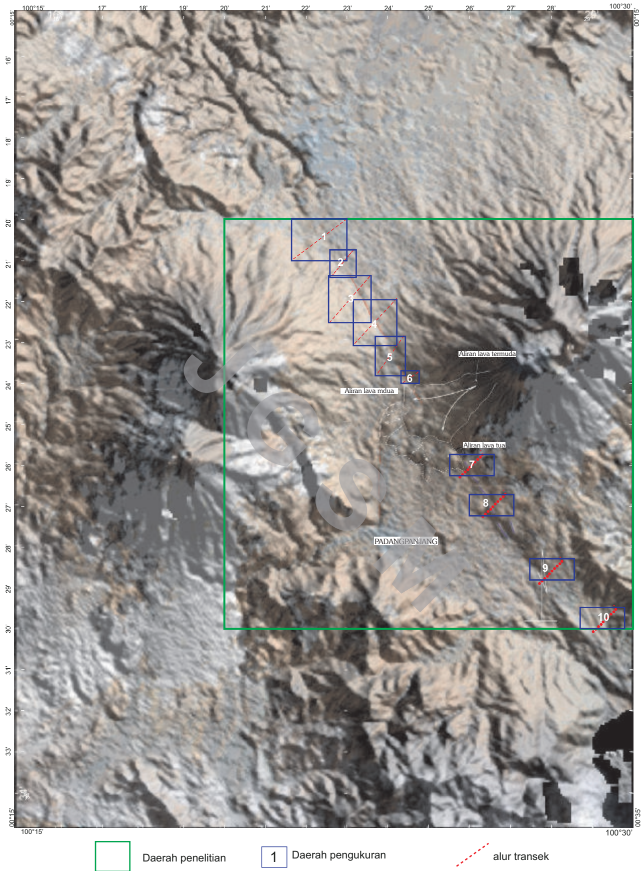
Gambar 7. Lokasi terpilih transek untuk identifikasi elemen morfostruktur daerah Padangpanjang dan sekitarnya.
