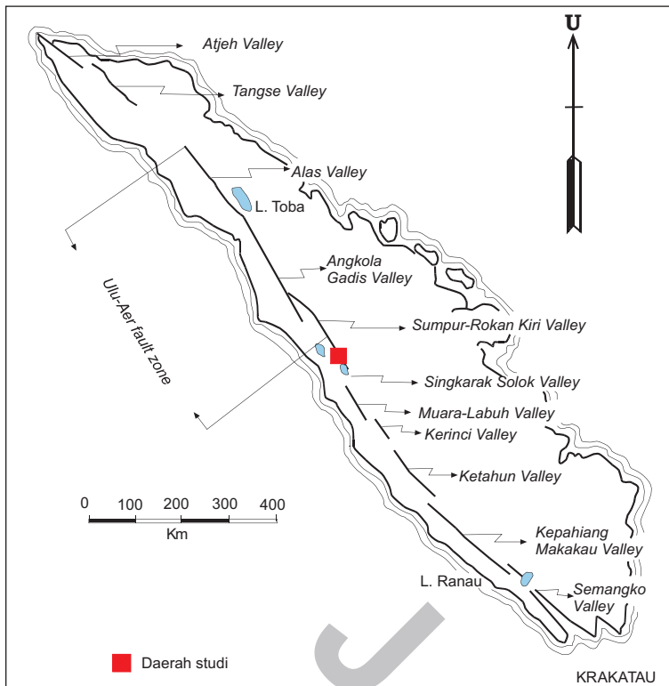
Gambar 1. Sesar besar Sumatera atau Zona Sesar Semangko (diambil dari Katili dan Hehuwat, 1967;h.7; kompilasi dari Durham, 1940; Westerveld, 1953 dan Klomppe, 1958).
