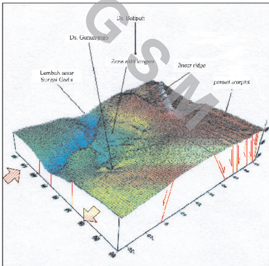
Gambar 13. Pandangan tiga dimensi bentuk lahan tektonik di sekitar Desa Gunungrajo-Batipuh, akibat pengaruh sesar Sumatera.
