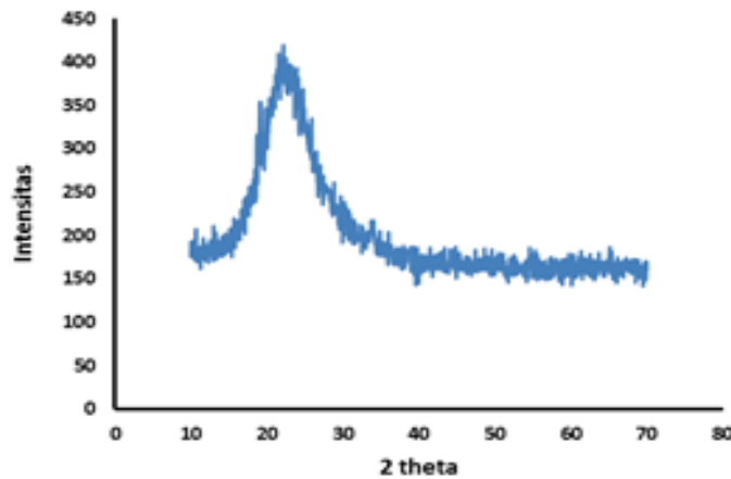
Gambar 2. Pola difraksi SiO 2 hasil sintesis
