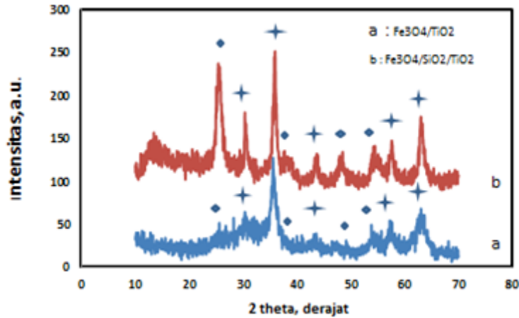
Gambar 1. Pola difraksi Fe 3 O 4 /TiO 2 dan Fe 3 O 4 /SiO 2 /TiO 2 hasil sintesis (◆ TiO 2 ; ★ Fe 3 O 4 )
