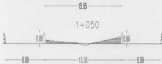
Gambar 5. Normalisasi Alternatif 1 Kala Ulang Q_{50} Sumber: Hasil Analisis
