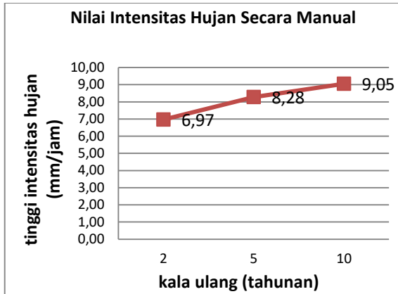
Gambar 10. Grafik intensitas hujan rancangan dengan analisis Manual
