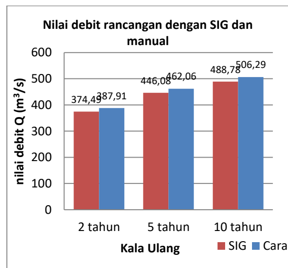
Gambar 16. Grafik perbandingan nilai debit rancangan dengan SIG dan Manual
