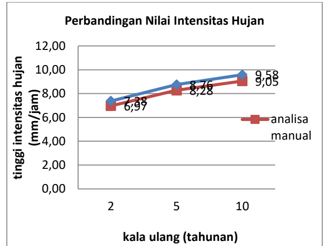
Gambar 11. Grafik perbandingan intensitas hujan rancangan dengan SIG dan manual
