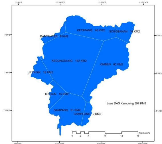
Gambar 8. Luas pengaruh curah hujan polygon Thiessen dengan SIG
