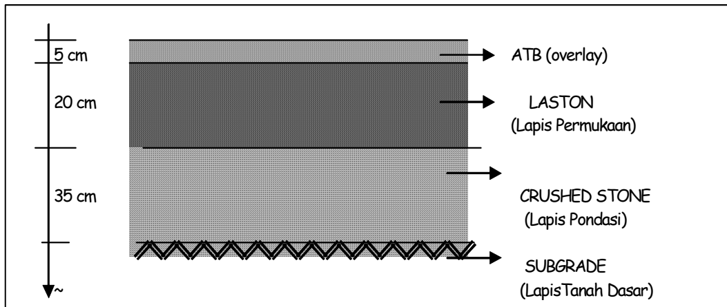
Gambar 1. Struktur perkerasan eksisting
