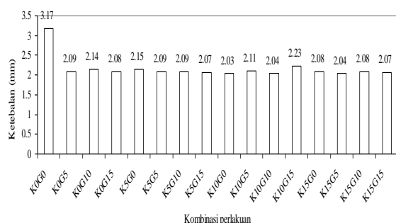
Gambar 2. Grafik hasil pengujian terhadap ketebalan pada semua perlakuan.
