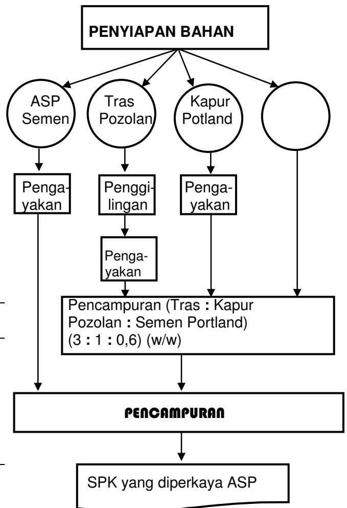
Gambar 1. Diagram Alir Pembuatan SPK yang diperkaya ASP
