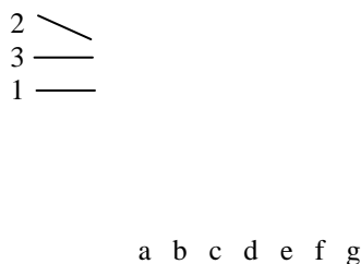
Gambar 2. Elektroforegram gel agarosa plasmid pUC19 hasil uji aktivitas protein fraksi pengendapan (F) terhadap DNA superkoil. (a) Kontrol (plasmid pUC19 tanpa pemberian ekstrak), (b) pUC19 setelah pemberian 2 \mu g protein ekstrak gubal, (c) pUC19 setelah pemberian 2 \mu g F-20, (d) F-40, (e) F-60, (f) F-80 dan (g) F-100. Aktivitas ditandai dengan penipisan pita (1) DNA superkoil, penebalan pita (2) DNA nick circular dan munculnya pita (3) DNA linier.
