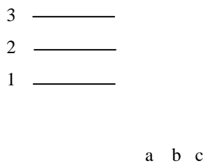
Gambar 1. Elektroforegram gel agarosa plasmid pUC19. (a) plasmid pUC19, terdapat 3 pita yaitu (1) pita plasmid bentuk superkoil, (2) bentuk nick circular dan (3) kontaminan kromosom E. coli , (b) pUC19 terdigesti oleh enzim EcoR1 , (c) marker Lambda- HindIII .
