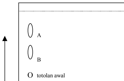
Gambar 1. Hasil pemisahan senyawa dengan fase diam selulosa dan fase gerak etanol – air ( 1:4 v/v)
