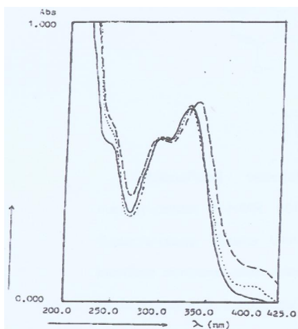
Gambar 5. Spektra flavonoid A1 dalam MeOH + AlCl 3 dan AlCl 3 + HCl --- = MeOH: 250, 300 s , 325 ..... = MeOH + AlCl 3 : 250, 300 s , 328 ..... = MeOH + AlCl 3 + HCl : 250, 300 s , 325
