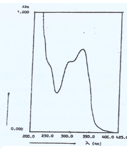
Gambar 6. Spektra hasil hidrolisis asam flavonoid dalam MeOH --- = MeOH : 250, 300 s , 325
