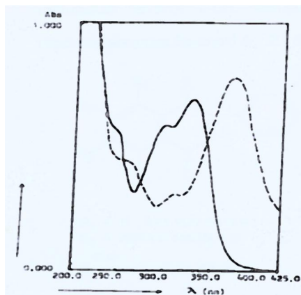
Gambar 3. Spektra flavonoid A1 dalam MeOH dan NaOH --- = MeOH : 250, 300 s , 325 .... = MeOH + NaOH : 267, 310 s , 375
