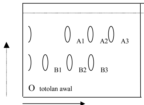
Gambar 2. Hasil pemisahan senyawa dengan dari kromatogram pada gambar 1. dengan gerak butanol – asam - air ( 4 : 1 : 5 )
