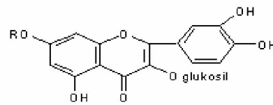
Gambar 9. Flavonoid pada bercak B2
