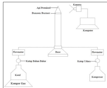
Gambar 1. Skema Instalasi
