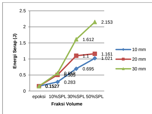
Gambar 7. Hubungan Rata-rata Energi Serap Vs Fraksi Volume Serat Pelepah Lontar
