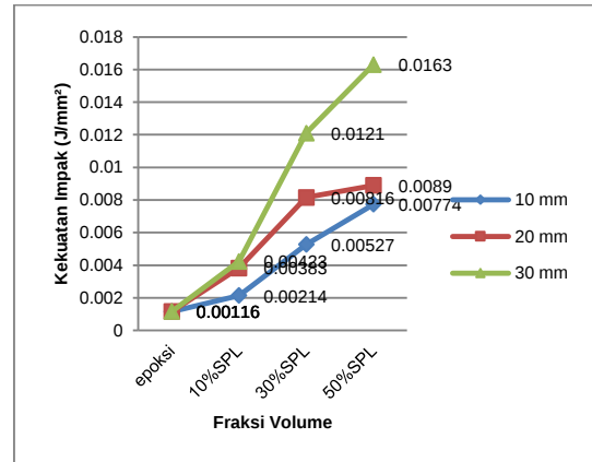
Gambar 8. Hubungan Rata-rata Kekuatan Impact Komposit Vs Fraksi Volume Serat Pelepah Lontar
