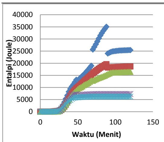
Gambar 5 Grafik hubungan antara waktu dengan entalpi gas pirolisis pada berbagai variasi temperatur
