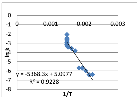
Gambar 6 Grafik hubungan antara 1/T dan \ln k pada temperatur 673 K ( kinetic rate lokal)
