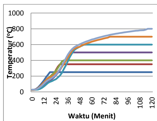
Gambar 3 Grafik Hubungan antara Waktu terhadap Temperatur Pirolisis
