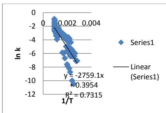
Gambar 7 Grafik hubungan 1/T dan \ln K untuk kinetic rate total.
