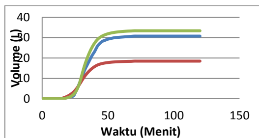
Gambar 8 Grafik Perbandingan Volume Gas Temperatur 673 K dengan Variasi Kinetik Rate
