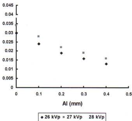
Gambar 5. Hasil Pengukuran HVL
