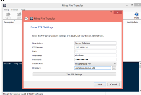
Gambar 6 Konfigurasi Aplikasi Fling
