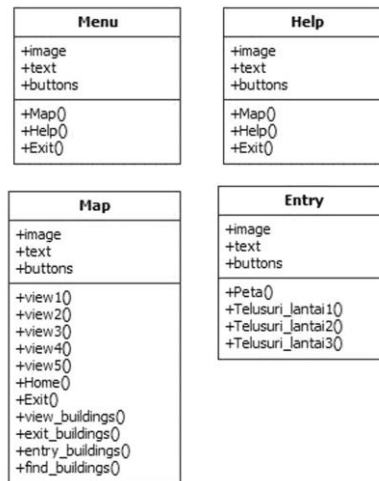
Gambar 4. Class Diagram Aplikasi Peta 3D UNIMA
