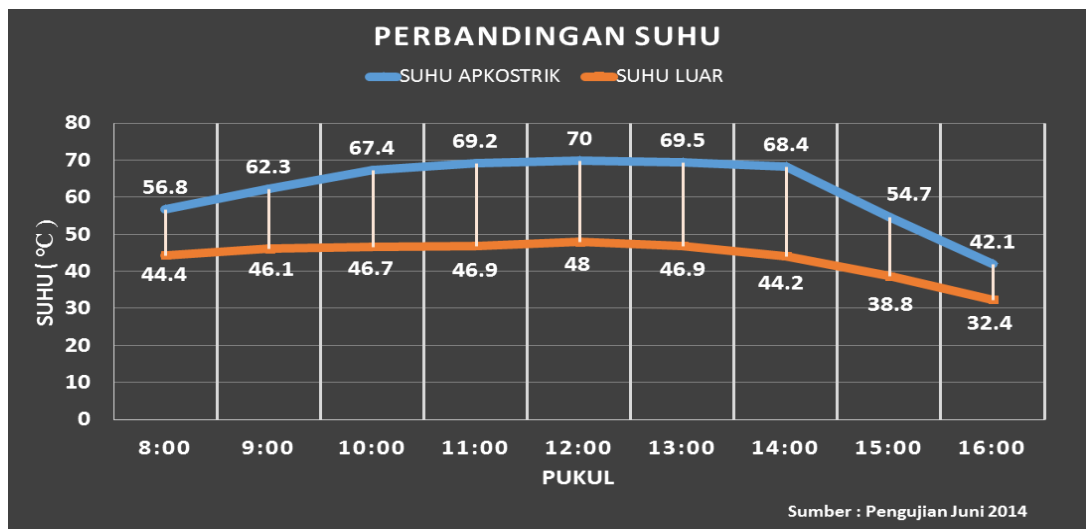
Gambar 4. Perbandingan Suhu Pengeringan Menggunakan APKOSTRIK dan Alami
