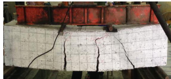
Gambar 9. Pola retak balok beton bertulangan bambu dengan kait jarak 10 cm
