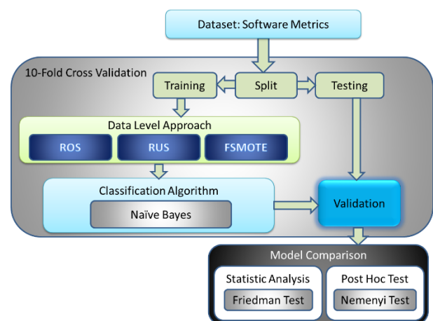
Gambar 1 Kerangka Kerja Model yang Diusulkan
