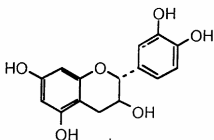
Gambar 1. Struktur Katekin
