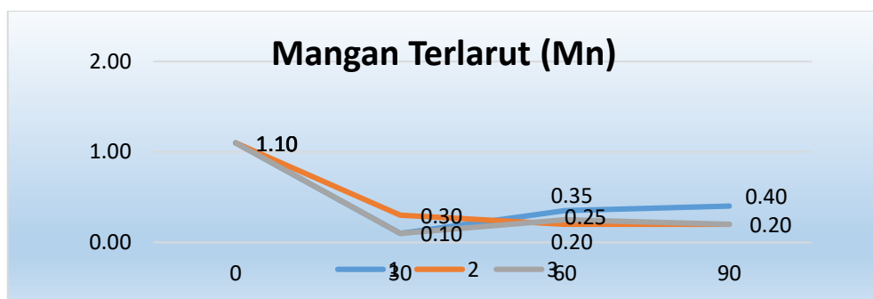
Gambar 2. Grafik Hasil Proses Filtrasi Mangan (Mn)
