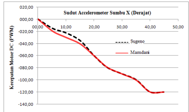
Gambar 18. Hasil pengujian gerak mundur dan belok kanan pada sumbu X
