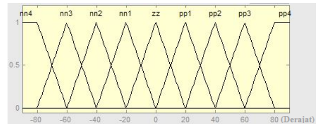
Gambar 3. Variabel input accelerometer sumbu Y
