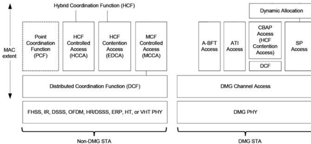
Gambar 3. Arsitektur MAC 802.11 [17, 18]
