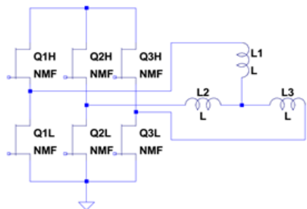
Gambar 1. Skematik motor DC Brushless Tiga Fasa
