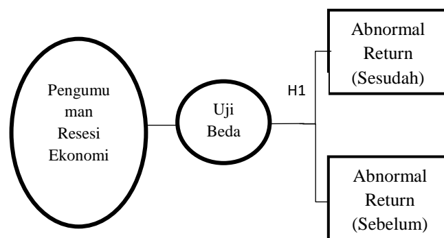
Gambar 2. Kerangka Pemikiran Teoritis Skema 1
