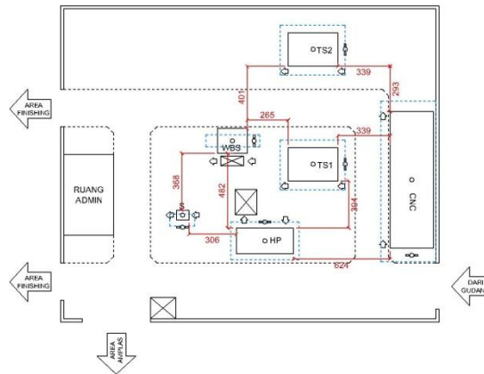
Gambar 4. Tata Letak Alternatif-2
