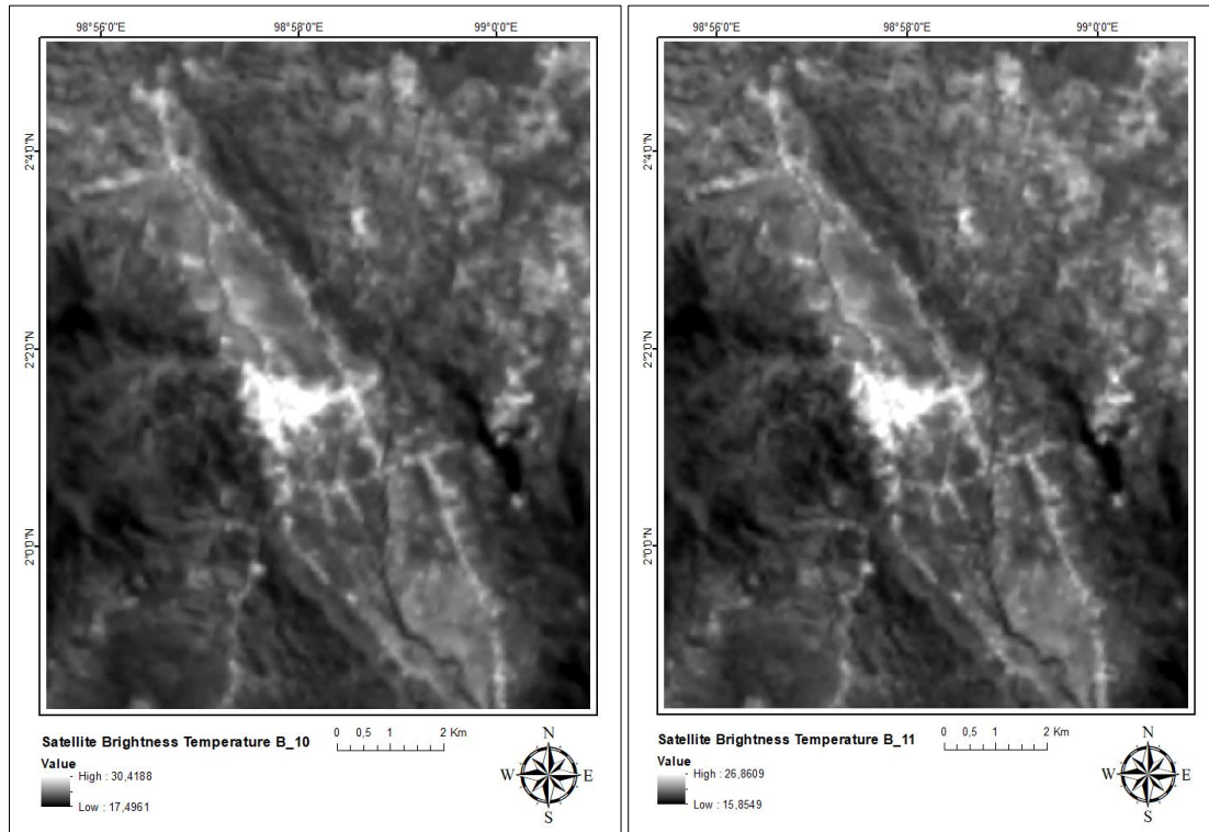
Gambar 4. Satellite Brightness Temperature Band 10 (kiri) dan Band 11 (kanan).
