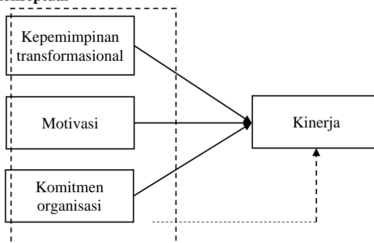
Gambar 1 Kerangka Konseptual
