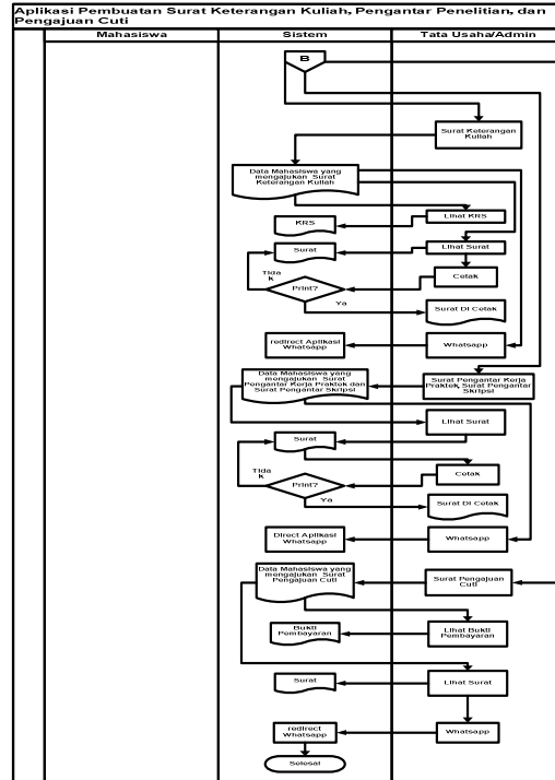
Gambar 2. Flowchart Pembuatan Aplikasi
