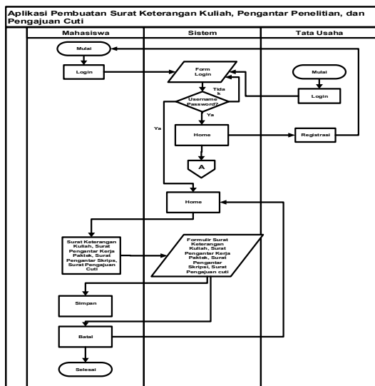
Gambar 1. Flowchart Usulan Aplikasi
