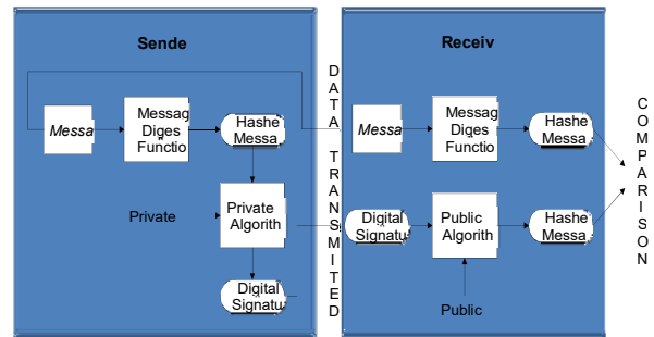
Gambar 1 Skema Tanda Tangan Digital
