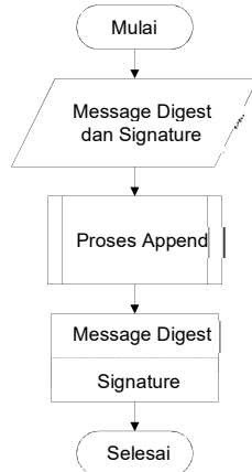
Gambar 10 Flowchart Penggabungan Pesan dan Digital Signature
