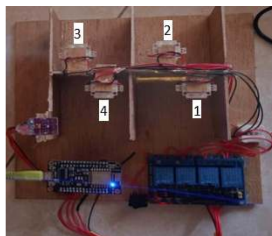
Gambar 7. Prototype Kontrol Penerangan Ruangan
