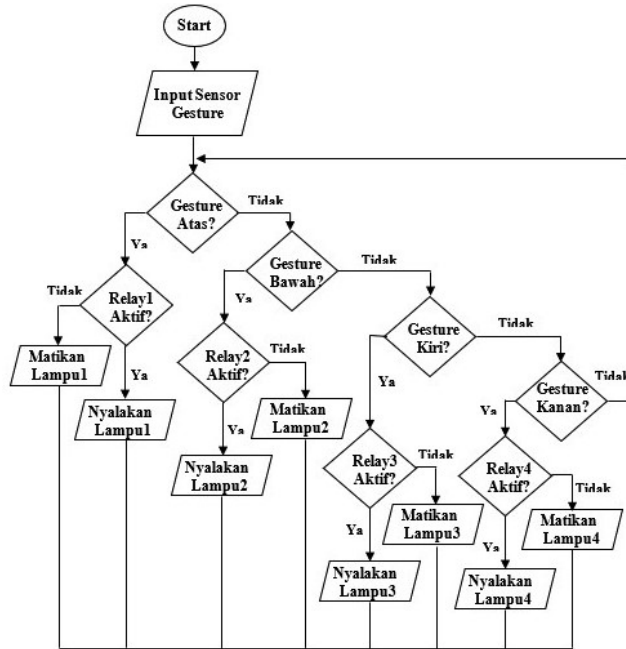
Gambar 2. Flowchart Penerangan Ruangan
