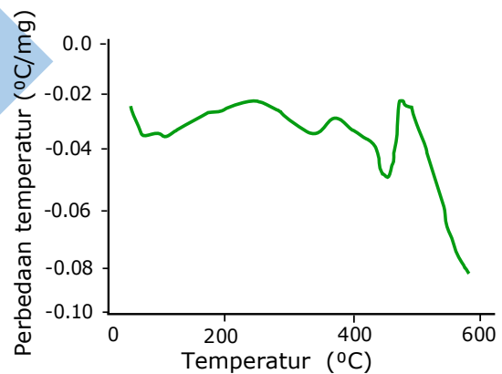
Gambar 6. Kurva DTA membran poliuretan
