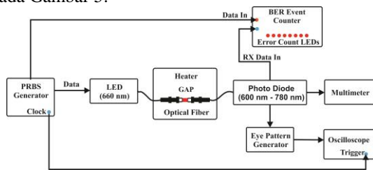
Gambar 5. Blok Diagram Konfigurasi Eksperimen
