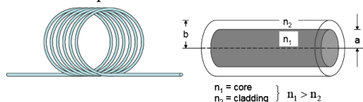
Gambar 2. Struktur POF [8]
