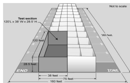
Gambar 2. Rangka Pondasi pontoon Sumber: http://www.wsdot.wa.gov.jpg .
