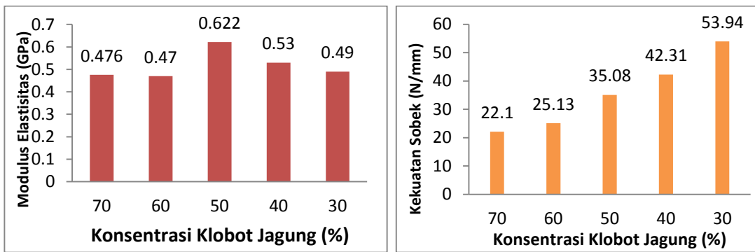
Gambar 3 (a) Perbandingan modulus elastisitas biokomposit (b) perbandingan kekuatan sobek biokomposit
