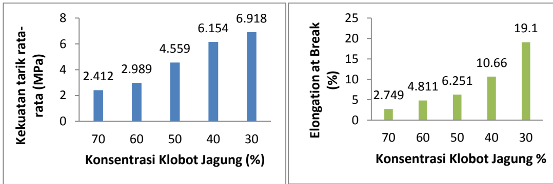
Gambar 2 (a) Perbandingan kekuatan tarik biokomposit (b) Perbandingan elongasi biokomposit
