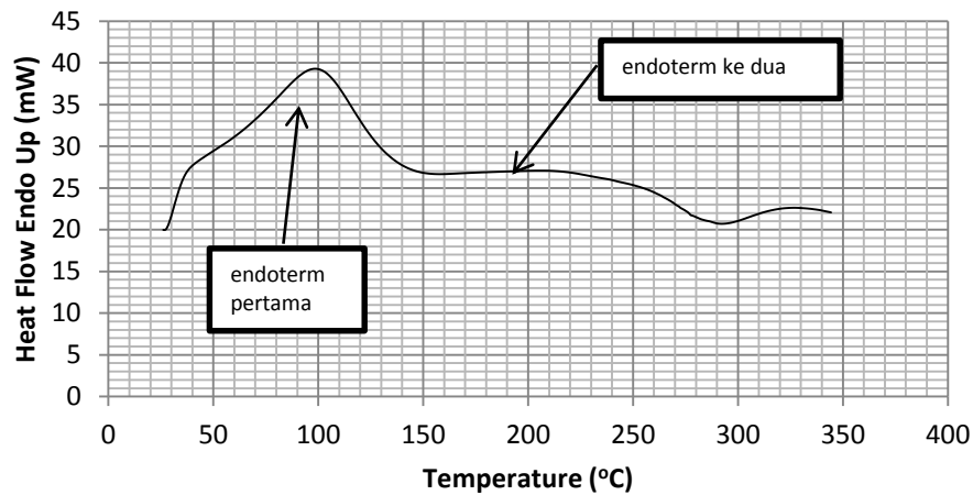
Gambar 1 Hasil uji DSC klobot jagung
