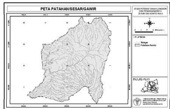
Gambar 6. Peta Patahan/Sesar/Gawir.
