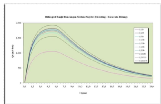
Gambar 3.2 hidrograf banjir rancangan HSS Snyder (Eksisting-Rerata Hitung)
