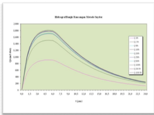
Gambar 3.9 hidrograf banjir rancangan HSS Snyder (Kagan-Rodda-Polygon Thiessen)
