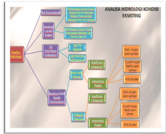
Gambar 3.1. Bagan Alir perhitungan Hidrologi kondisi eksisting
