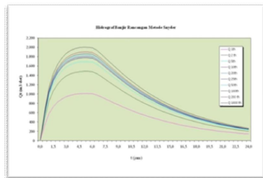
Gambar 3.8 hidrograf banjir rancangan HSS Snyder (Kagan-Rodda-Rerata Hitung)
