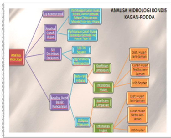
Gambar 3.7. Bagan Alir perhitungan Hidrologi kondisi Kagan-Rodda
