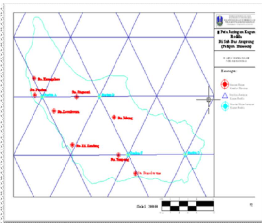
Gambar 3.6. Peta Jaringan Kagan Rodda (Poligon Thiessen)
