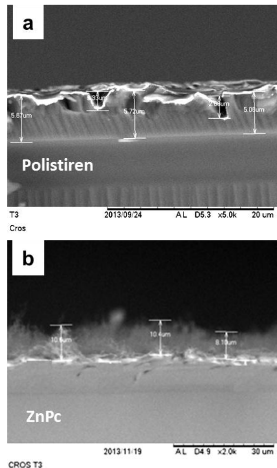
Gambar 1. Ketebalan Lapisan Hasil Karakterisasi SEM (a) ZnPc, (b) Polistiren
