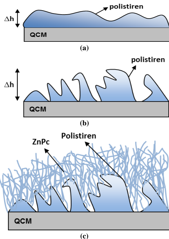
Gambar 3. Ilustrasi Ketebalan Lapisan dengan Permukaan Berbeda (a) Lapisan Polistiren dengan Permukaan Padat (b) Permukaan Berongga (c) ZnPc di atas Permukaan Polistiren
