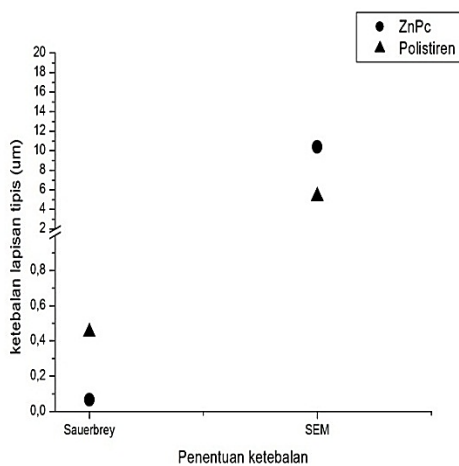
Gambar 2. Grafik Perbandingan Ketebalan Lapisan Hasil Pengukuran SEM dan Persamaan Sauerbrey
