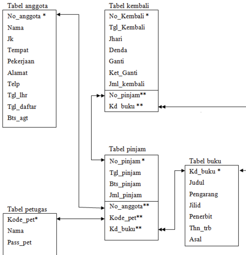
Gambar 2. Bentuk Normal Ketiga (3NF)
