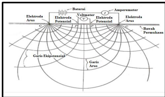
Gambar 4 Garis arus listrik dan medan potensial yang timbul karena adanya dua sumber arus listrik (Todd, 1959).
