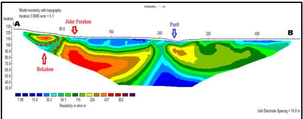
Gambar 10 Dugaan keberadaan rekahan pada Lintasan 2
