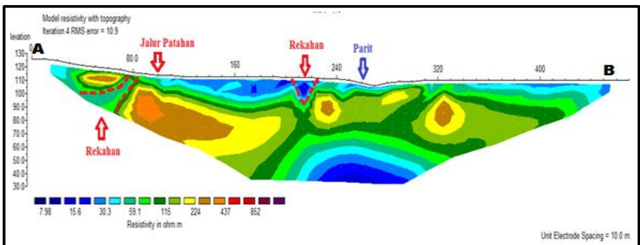
Gambar 11 Dugaan keberadaan rekahan pada Lintasan 3
