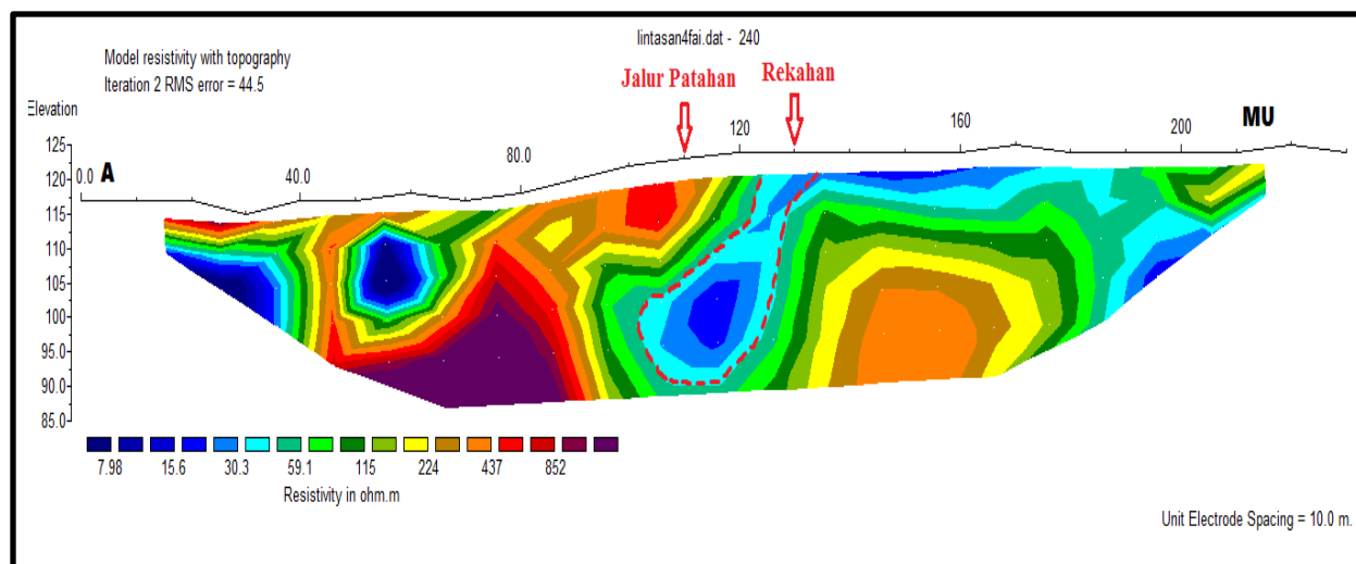
Gambar 12 Dugaan keberadaan rekahan pada Lintasan 4
