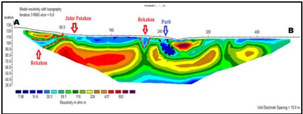
Gambar 9 Dugaan keberadaan rekahan pada Lintasan 1
