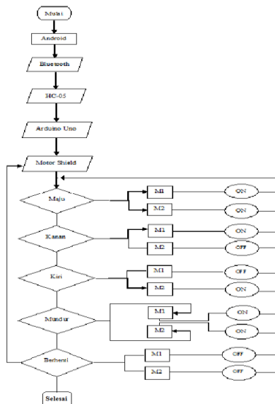
Gambar 3.7 : Perancangan perangkat lunak
