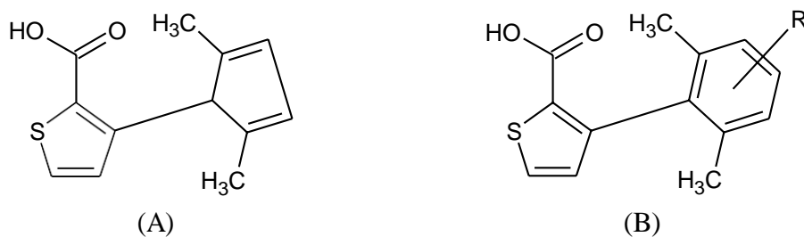
Gambar 1. Senyawa Pyrrothiogatain (A) yang digunakan sebagai kontrol positif dan senyawa turunannya yang digunakan sebagai derivat utama (B)
