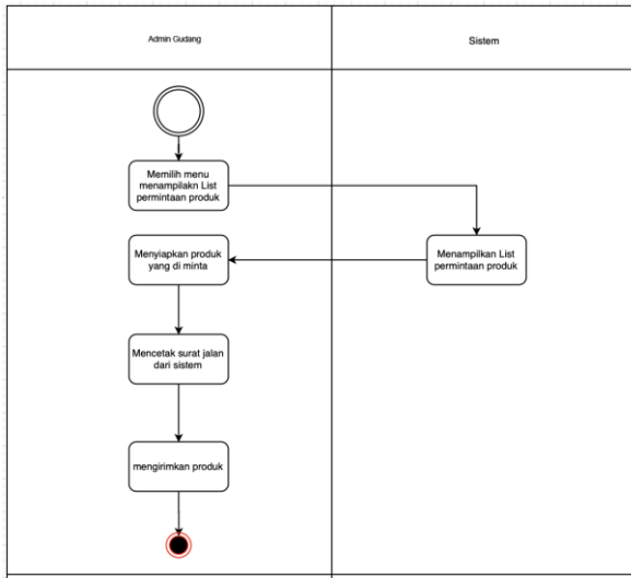
Gambar 4: Activity Diagram Produk Keluar
