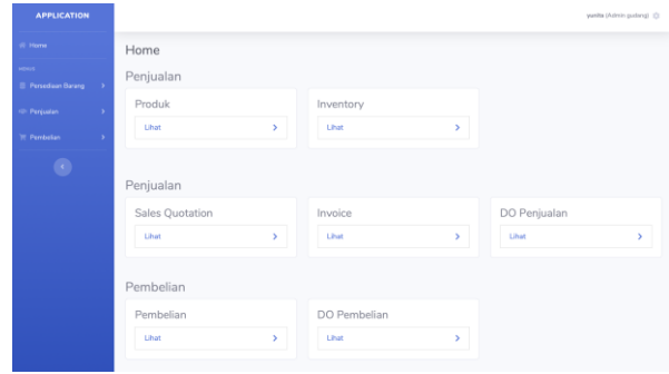
Gambar 13: Tampilan Aplikasi
