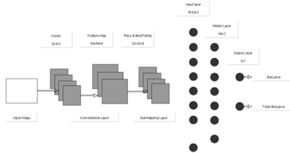
Gambar 4. Arsitektur CNN
