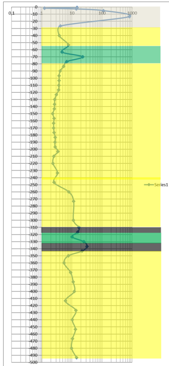
Gambar 8. Profil Inversi 1D titik pengukuran 3 dan interpretasi shallow Hydrocarbon pada formasi Wonocolo
