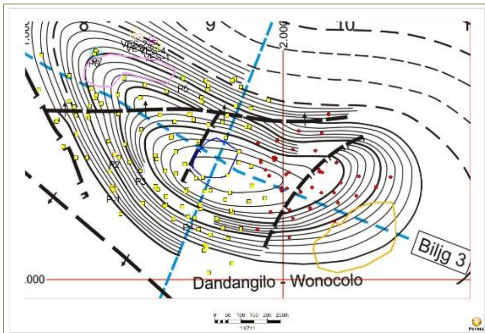
Gambar 5. Peta top struktur Formasi Wonocolo
