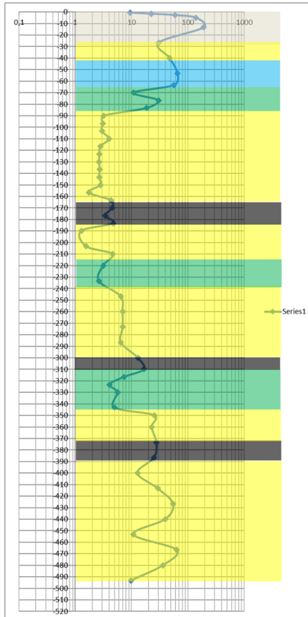
Gambar 9. Profil Inversi 1D titik pengukuran 2 dan interpretasi shallow Hydrocarbon pada formasi Wonocolo
