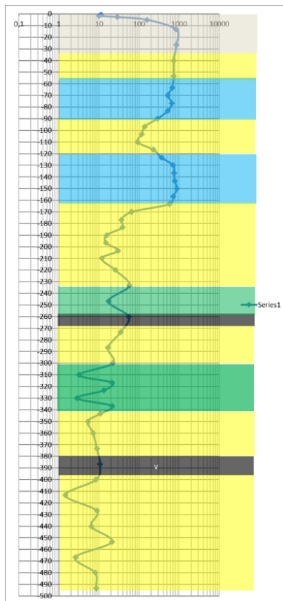
Gambar 7. Profil Inversi 1D titik pengukuran 1 dan interpretasi shallow Hydrocarbon pada formasi Wonocolo
