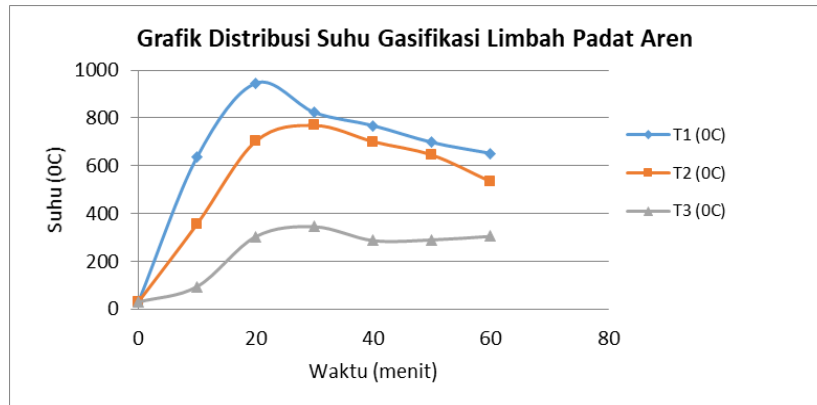
Gambar 3. Distribusi Suhu Gasifikasi Limbah Padat Aren
